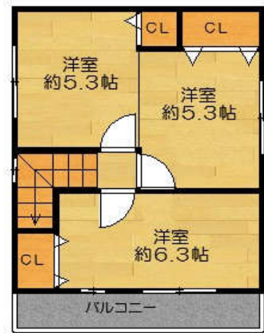
3階平面図
